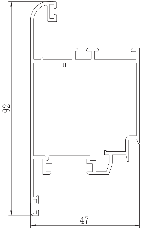
HOJA PUERTA APERTURA EXTERIOR ZX-4023
