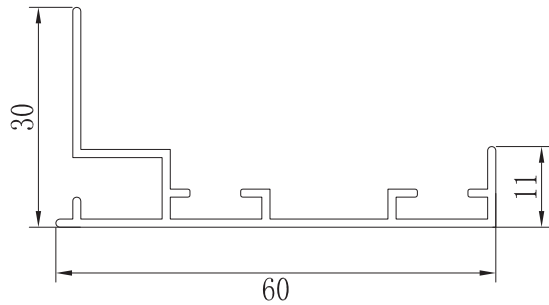
FORRO RECTO 60 ZX-02
