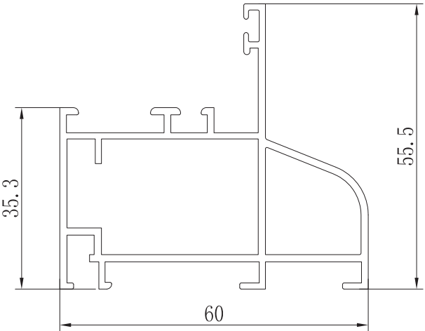
MARCO DE PUERTA 60 ZX-4031
