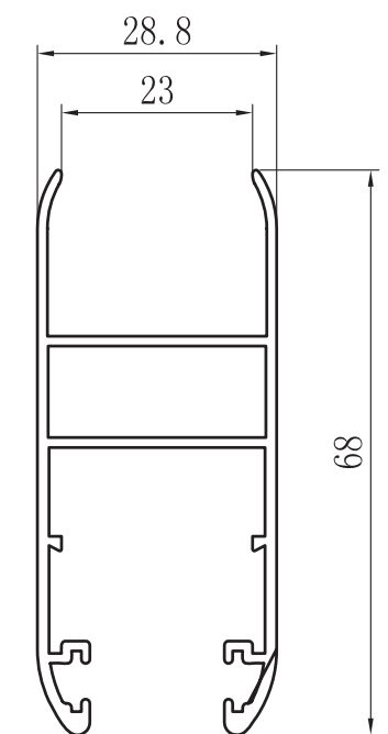
HOJA PERIMETRAL EVO 68 ZX-6302
