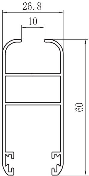
HOJA PERIMETRAL 60 (VIDRIO10) ZX-6002
