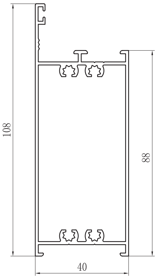
ZOCALO ZX-4001 B
