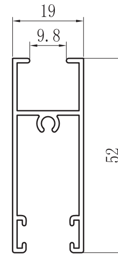
CASACA (VIDRIO 10) ZX-6204D
