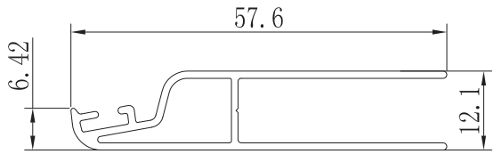
CIERRE COMPENSADOR MALLORQUINA ZX-06
