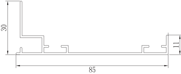
FORRO RECTO 85 ZX-03
