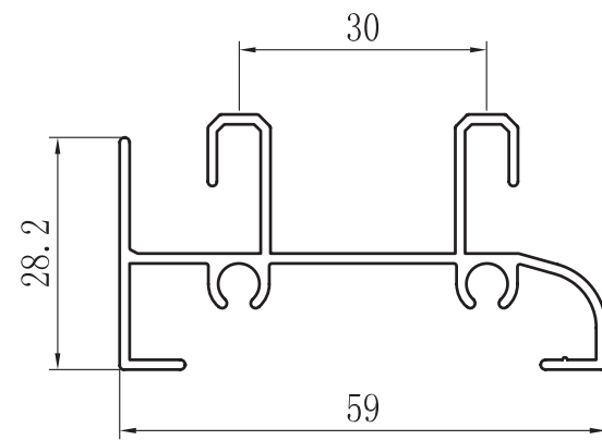
MARCO INFERIOR ZX-6202
