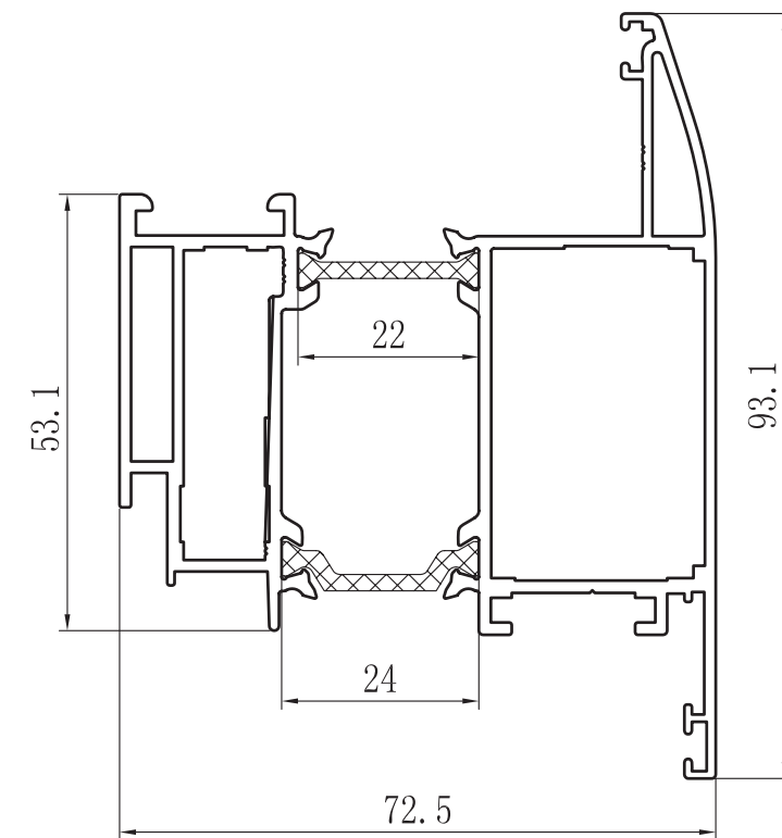
HOJA APERTURA EXTERIOR R.P.T. ZX-6503CD
