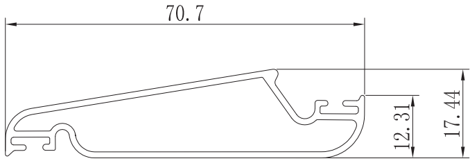
LAMA MOVIL MALLORQUINA ZX-05
