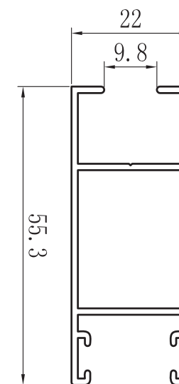
HOJA CIERRE (VIDRIO 10) ZX-6206D
