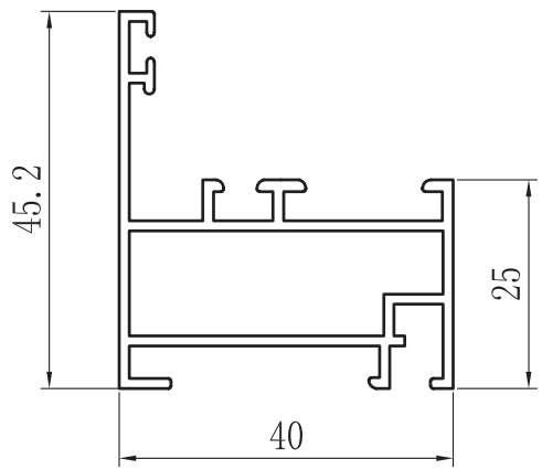
MARCO FIJO 40 ZX-4001
