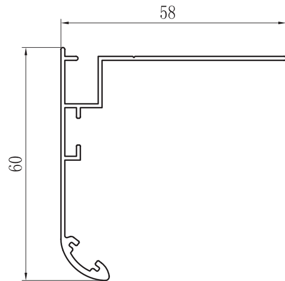
FORRO REDONDOS CON REGISTRO 60X58 ZX-6008
