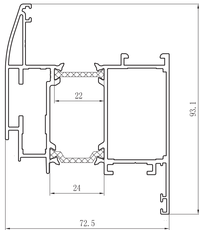
HOJA DE PUERTA R. P. T ZX-6513
