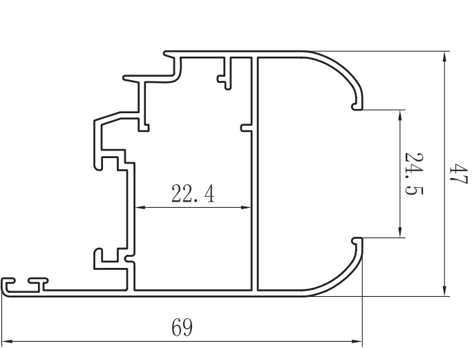
HOJA APERTURA EXTERIOR ZX-4013
