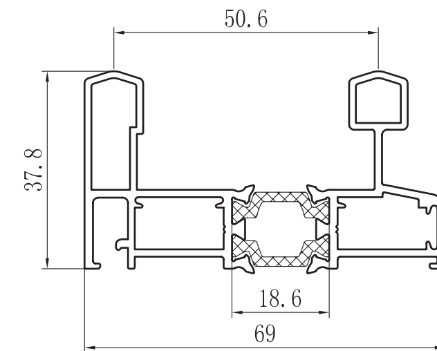
MARCO PERIMETRAL CERRADO 70 R.P.T. ZX-7001
