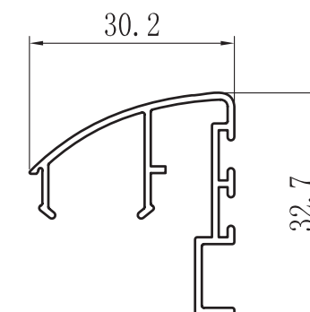
CLIP CRUCE EVO PEQUEÑO ZX-6303A
