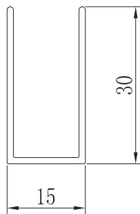
PERFIL "U" U15x30
