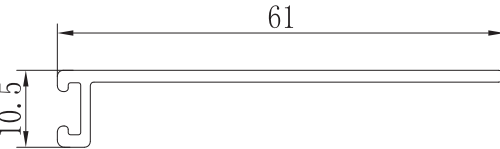
PERFIL LIMPIA PERSIANA ZX-04
