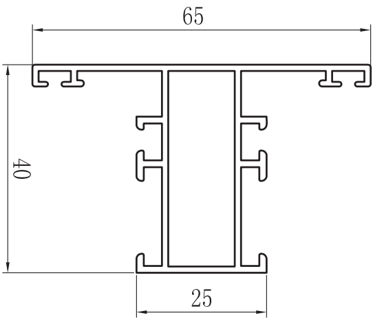
TRAVESAÑO DE 65 ZX-4002
