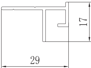
PERFIL REGISTRO 30 ZX-7012
