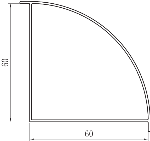
TUBOS ESQUINEROS DE 90° ZX-4005
