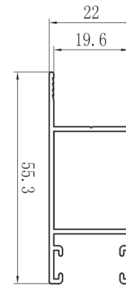
HOJA CIERRE ZX-6206
