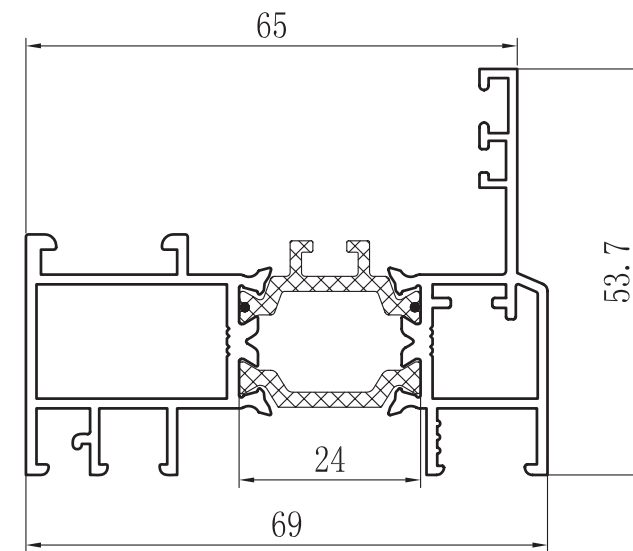
MARCO FIJO 70 R.P.T ZX-7003
