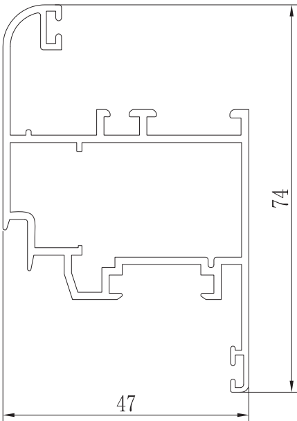
HOJA MEDIANA S/JUNQUILLO ZX-4043
