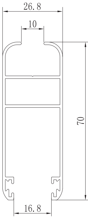
CLIP CRUCE ZX-6003
