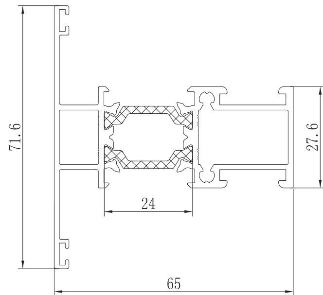
TRAVESAÑO 70 R.P.T. ZX-6512
