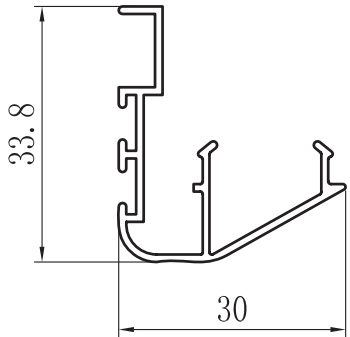
CLIP CRUCE ZX-6003
