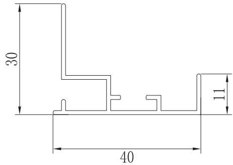
FORRO RECTO 40 ZX-01
