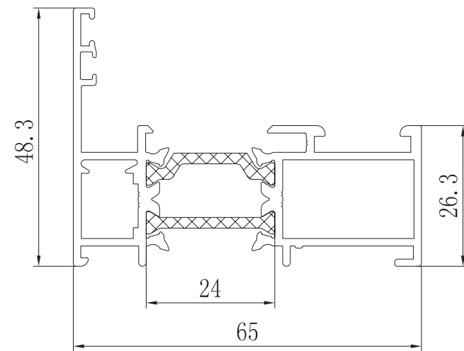
MARCO FIJO 65 RPT ZX-6501
