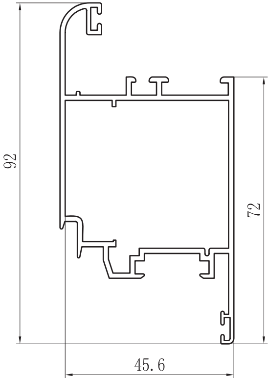
HOJA PUERTA ZX-4003B
