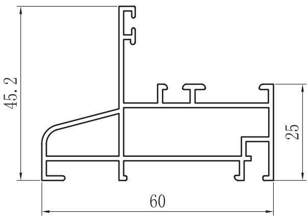
MARCO FIJO 60 ZX-4001A
