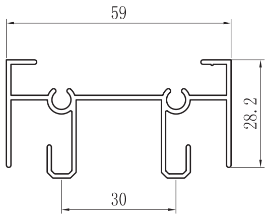
MARCO SUPERIOR ZX-6201
