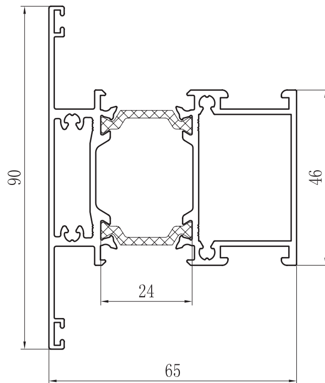
TRAVESAÑO 90 RPT ZX-6502
