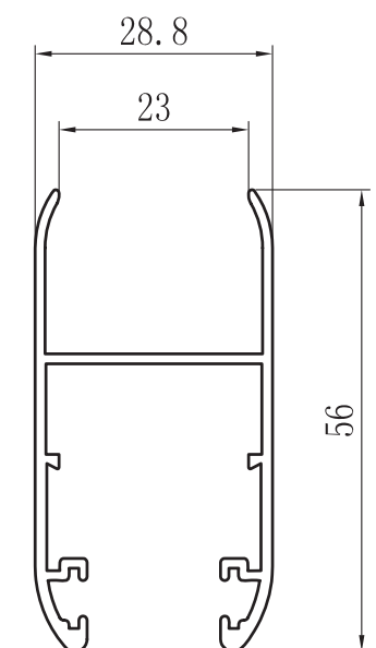
HOJA PERIMETRAL EVO 56 ZX-6302A
