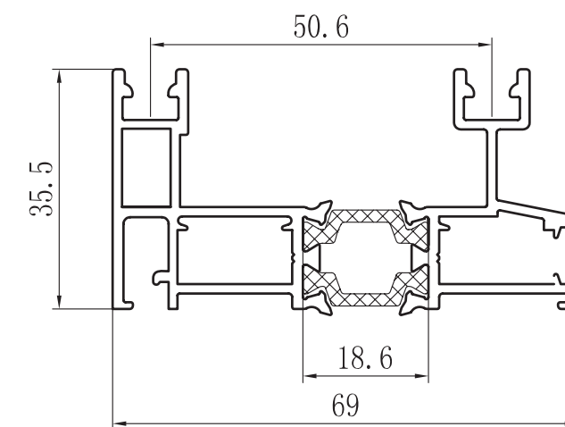
MARCO PERIMETRAL RIEL CLIPADO 70 R.P.T. ZX-7002
