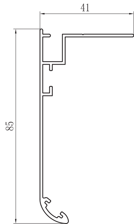
FORRO REDONDOS CON REGISTRO 85X41 ZX-6006
