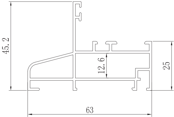
MARCO FIJO 63 ZX-4021
