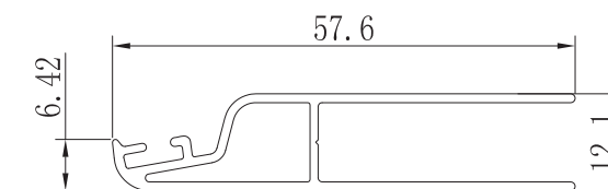
CIERRE COMPENSADOR MALLORQUINA ZX-06
