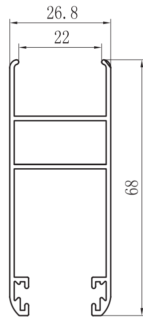
HOJA PERIMETRAL 70 (VIDRIO22) ZX-6002B
