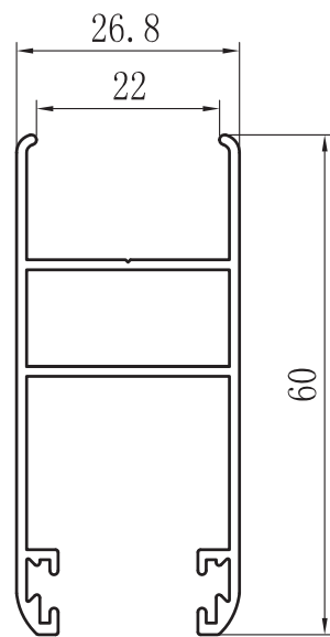
HOJA PERIMETRAL 60 (VIDRIO22) ZX-6002A
