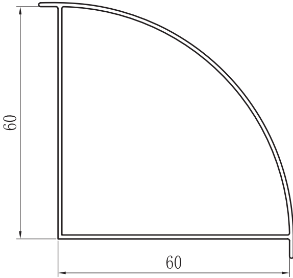
TUBOS ESQUINEROS DE 90° ZX-4005
