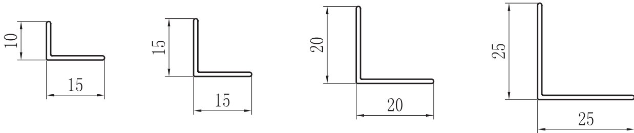
ANGULOS A15x10 ANGULOS A15x15 ANGULOS A20x20 ANGULOS A25x25
