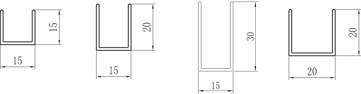
PERFIL "U" U15x15 PERFIL "U" U15x20 PERFIL "U" U15x30 PERFIL "U" U20x20
