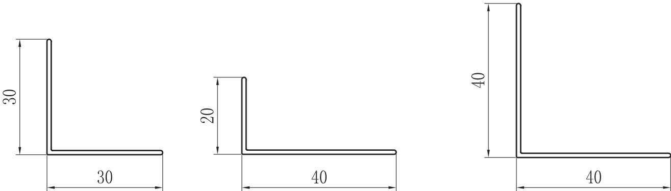
ANGULOS A30x30 ANGULOS A40x20 ANGULOS A40x40
