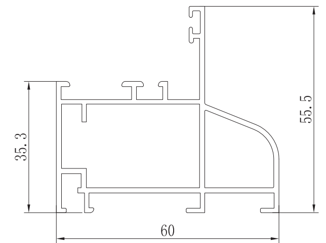
MARCO DE PUERTA 60 ZX-4031
