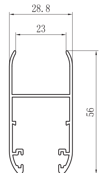
HOJA PERIMETRAL EVO 56 ZX-6302A
