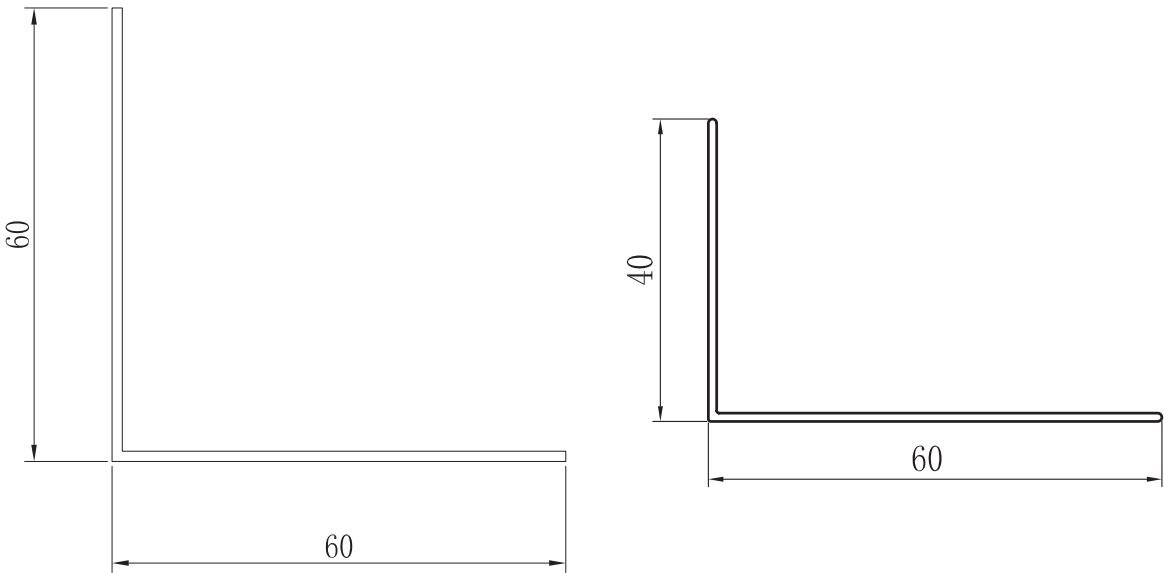
ANGULOS A60x60 ANGULOS A60x40
