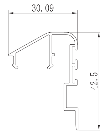
CLIP CRUCE GRANDE ZX-6003A
