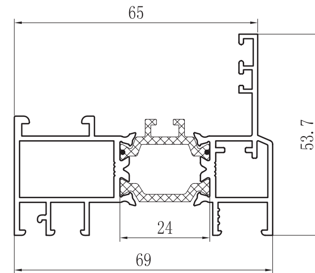
MARCO FIJO 70 R.P.T ZX-7003
